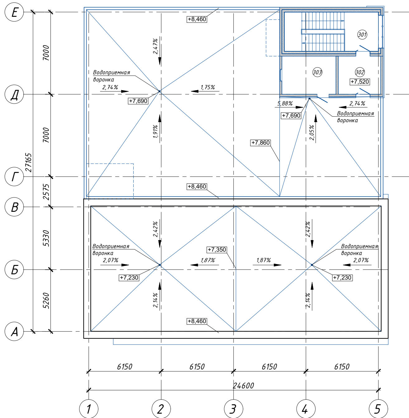
План кровли на отм. +7,820.
