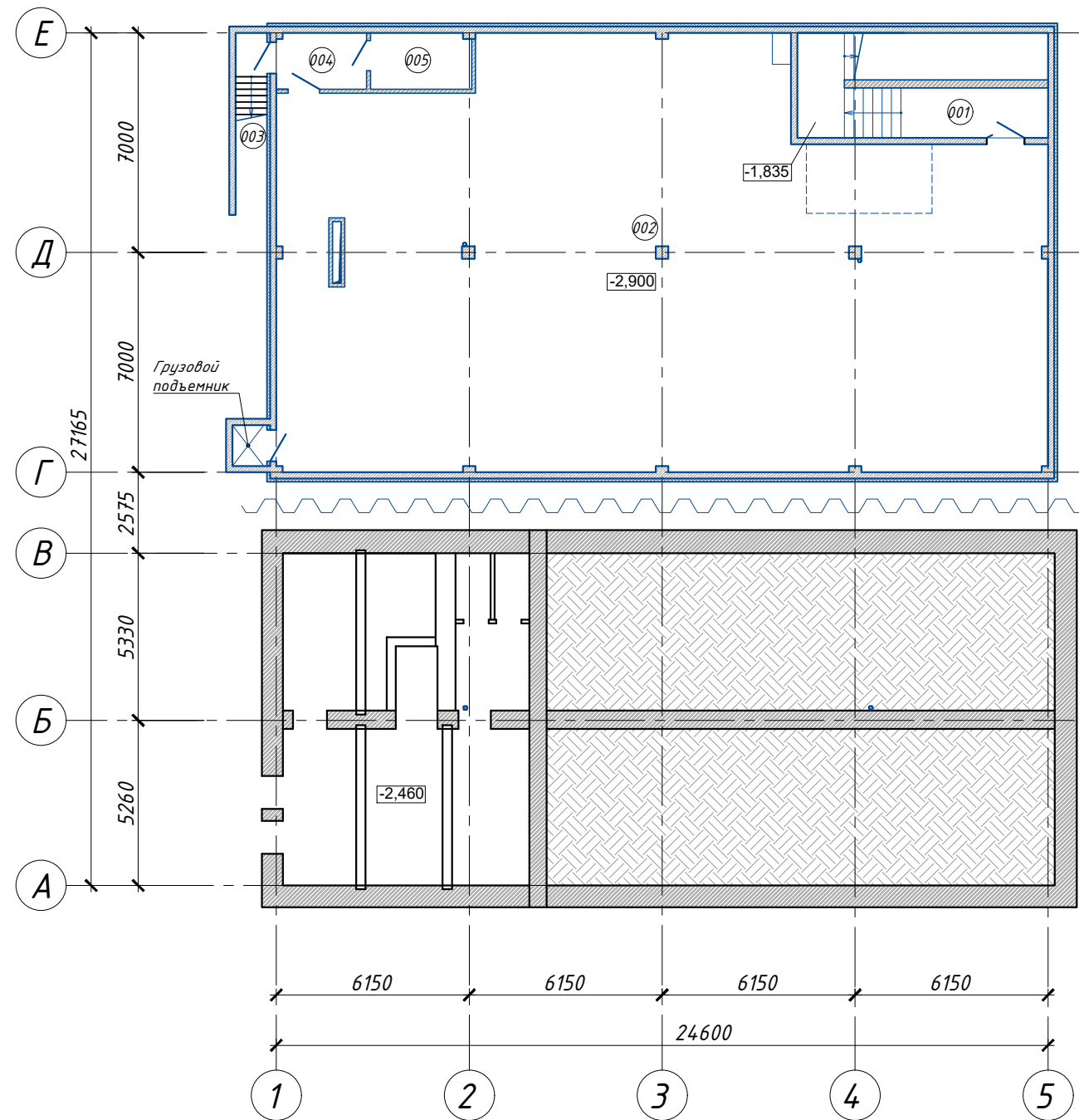
План подвала на отм. -2,900.
